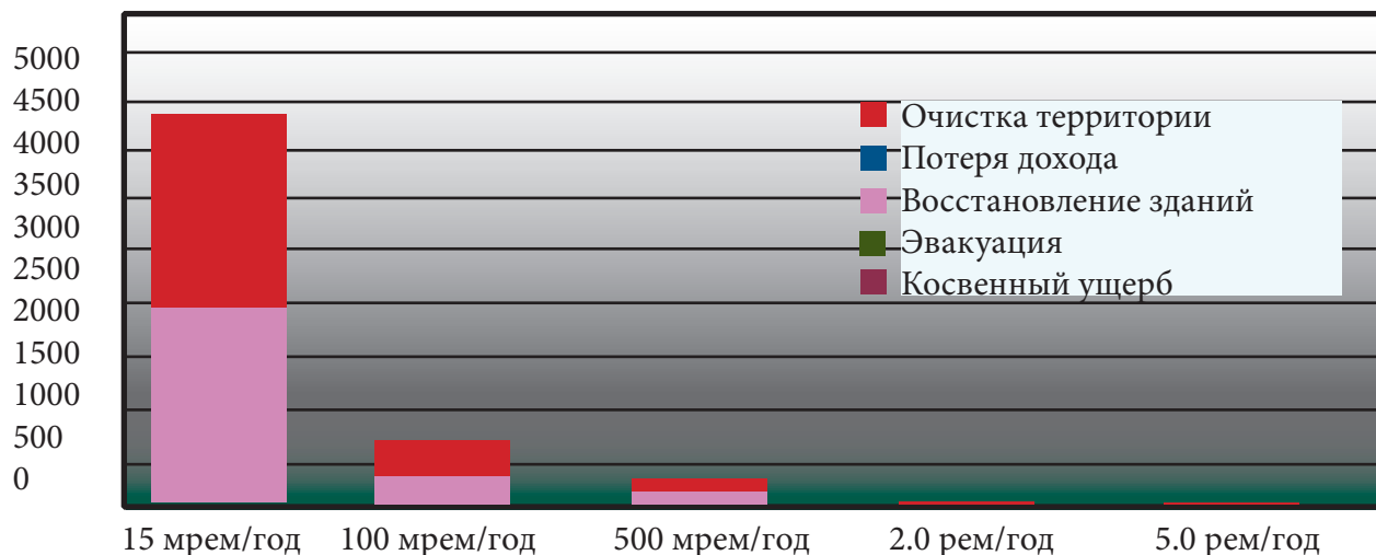
Рис. 6. Составляющие экономического ущерба в зависимости от критерия реабилитации территории для гипотетического сценария подрыва в Нью-Йорке «грязной бомбы» активностью 10000 Ки, содержащей 137 Cs (млрд долларов)
