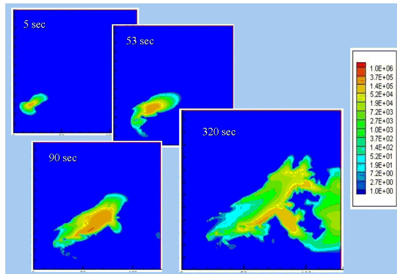
Рис. 2. Динамика изменения концентрации 241 Am в воздухе в случае подрыва взрывного устройства с включением в него радиоактивного источника для одного из вариантов городских условий, отн. ед.
