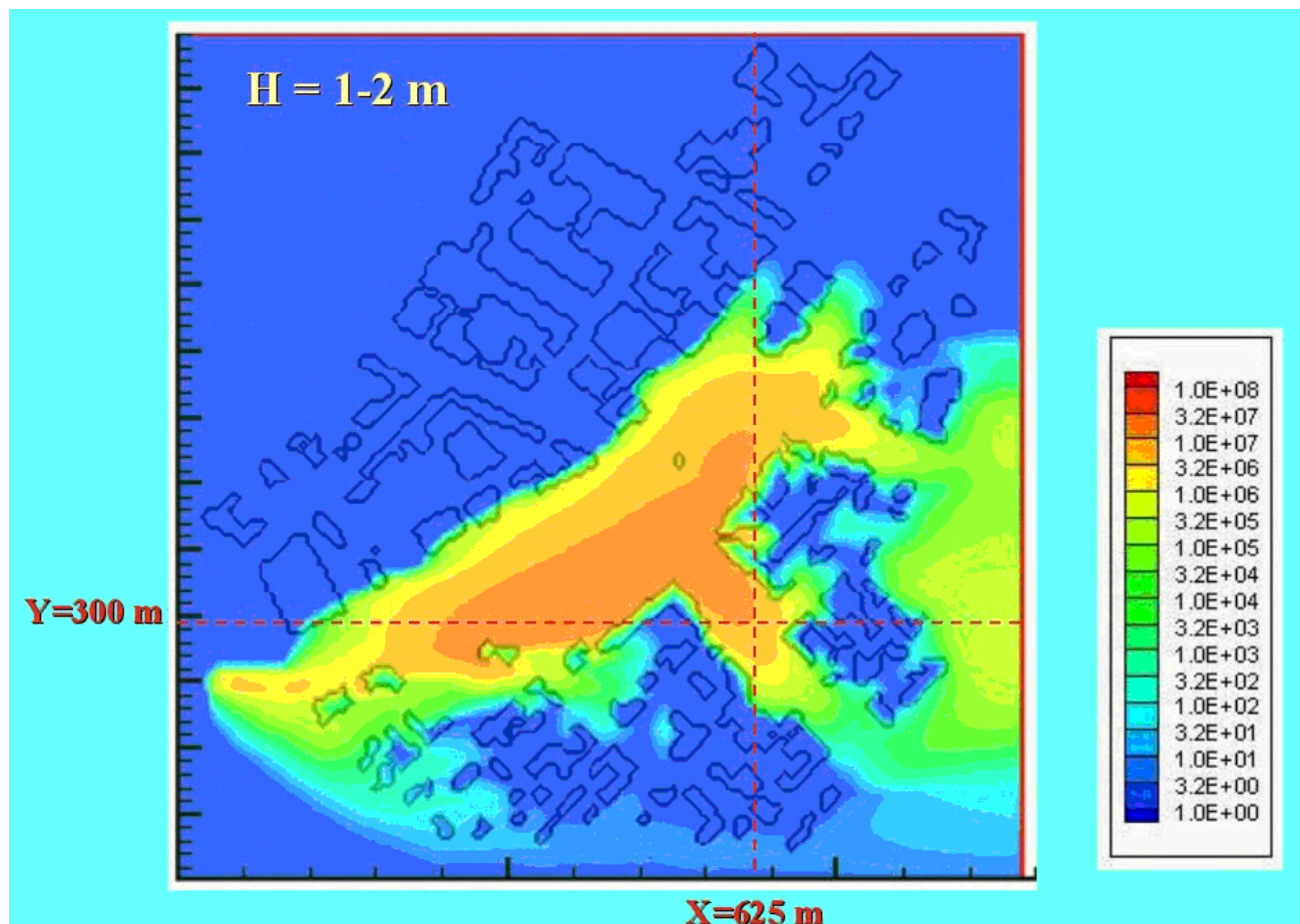
Рис. 3. Интеграл концентрации 241 Am в воздухе в случае подрыва взрывного устройства с включением в него радиоактивного источника для одного из вариантов городских условий, отн. ед.
