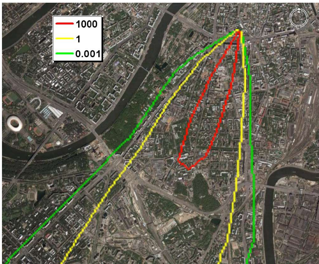
Рис. 4. Прогнозируемая плотность загрязнения местности на территории мегаполиса в случае диспергирования некоторого количества ^{137}\text{Cs} , Ки/км 2
