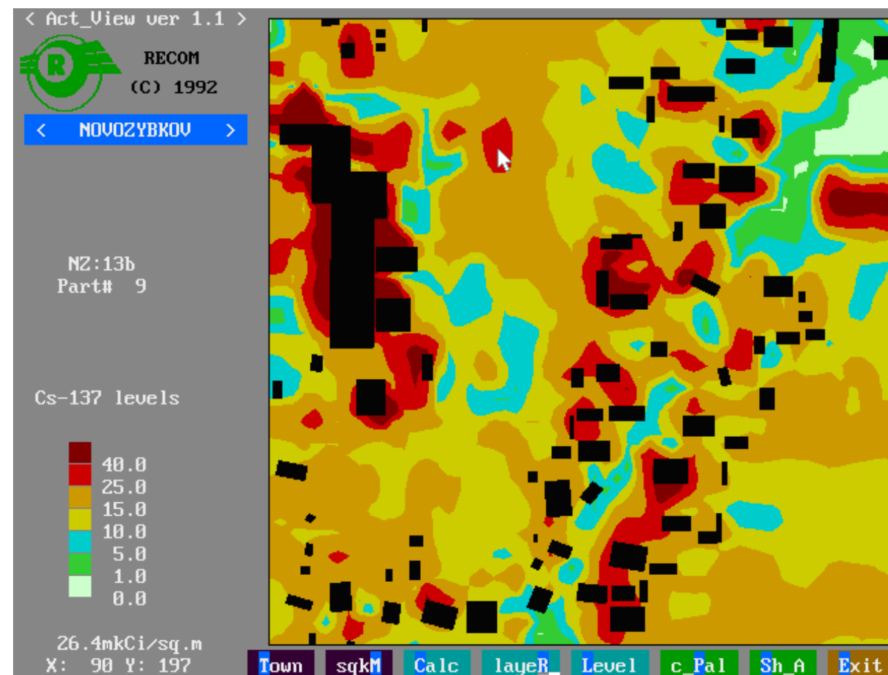
Рис. 5. Пример неравномерности радиоактивного загрязнения городской территории (Новозыбков, Брянская область, Российская Федерация)
